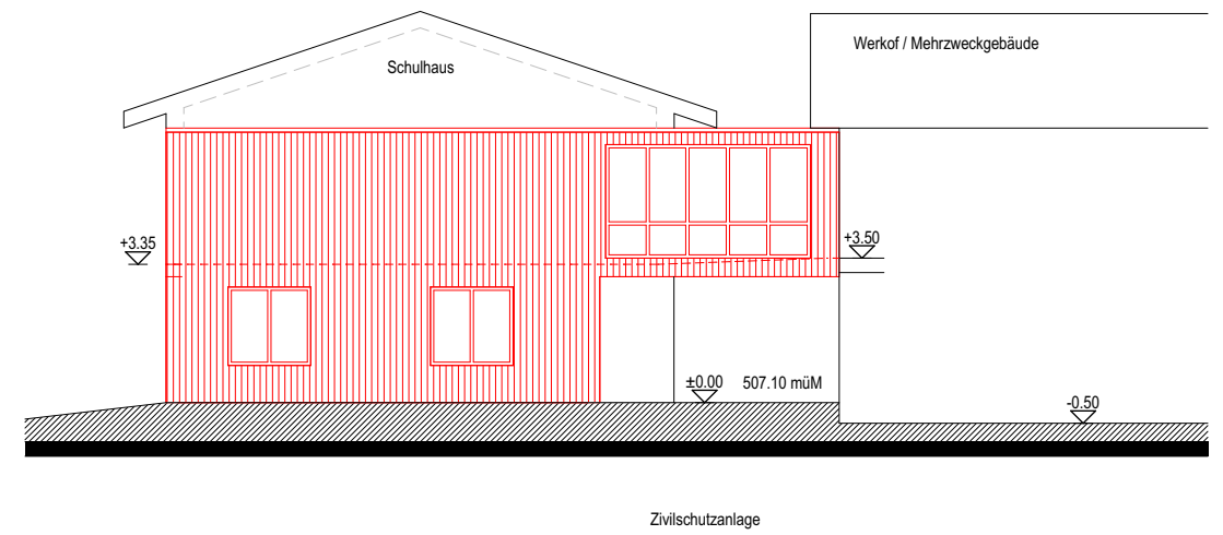
Ansicht Ost
