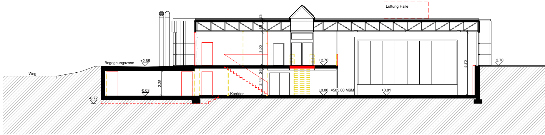
Schnitt B-B
