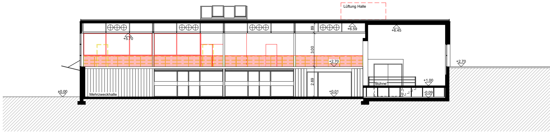
Schnitt A-A
